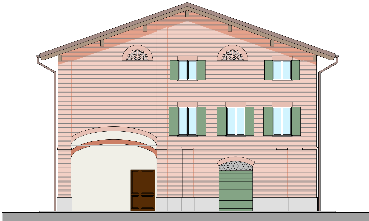
PROSPETTO EST
