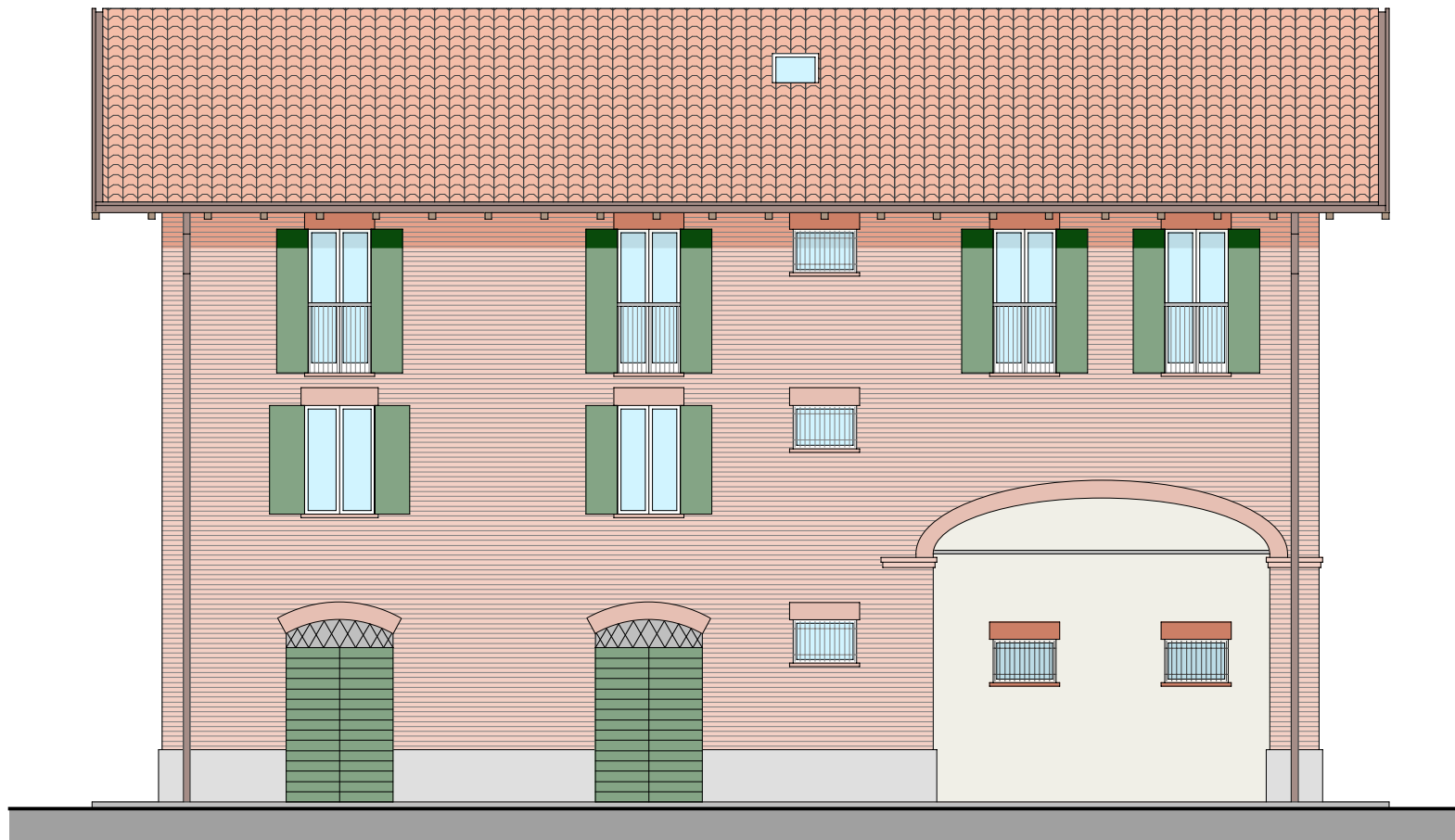
PROSPETTO SUD
